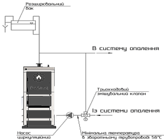
Рисунок 3- Схеми підключення котла до системи опалення
