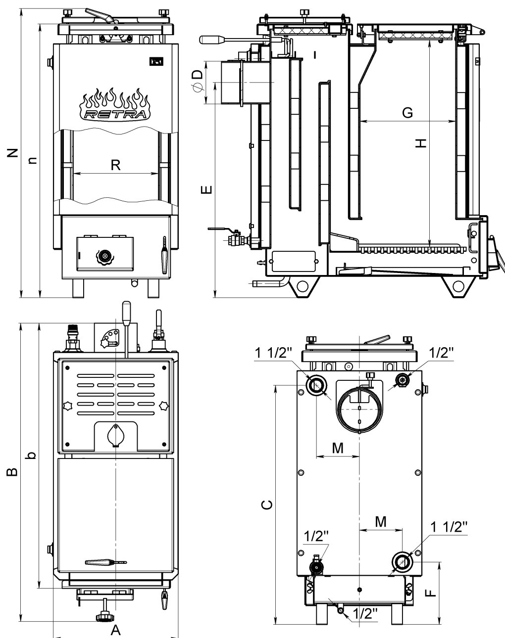
Рис.1а Габаритні та приєднувальні розміри котлів «Retra-6М» потужністю 16-40 кВт
