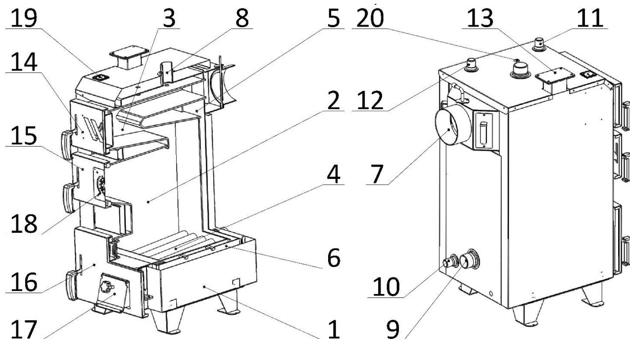
Рис. 1. Будова котлів серії WARMLINE ECO
