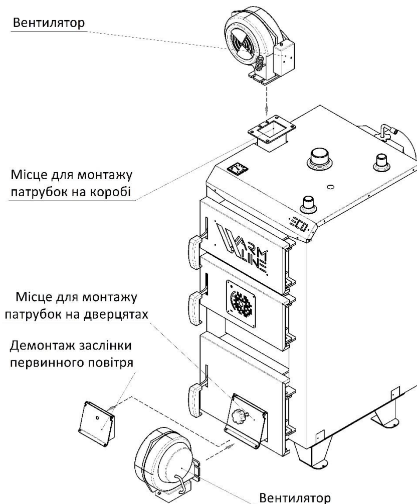
Рис. 7. Схема встановлення вентилятора
