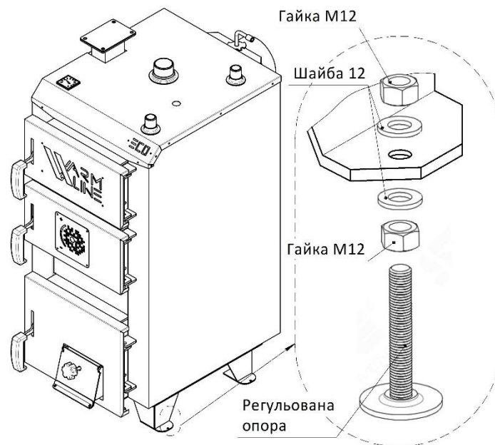
Рис. 4. Схема установки регулируемых опор
