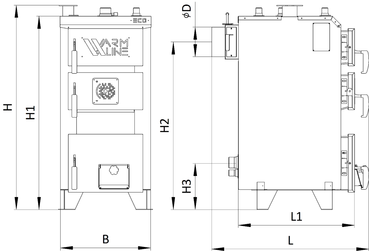
Рис. 2. Основні розміри котлів серії WARMLINE ECO
