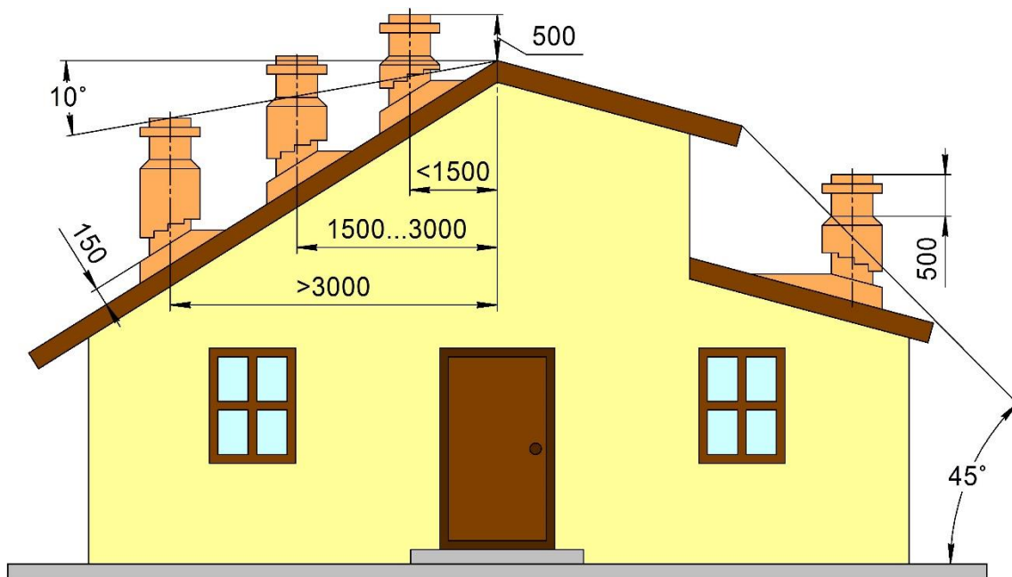
Рис. 5. Схема правильного вибору висоти димоходу над дахом
