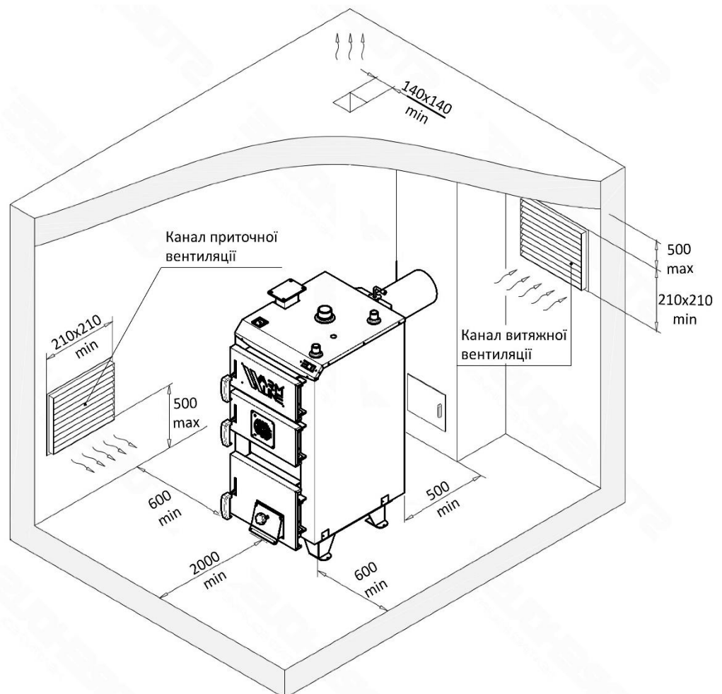
Рис. 3. Схема установки котла в приміщенні котельні
