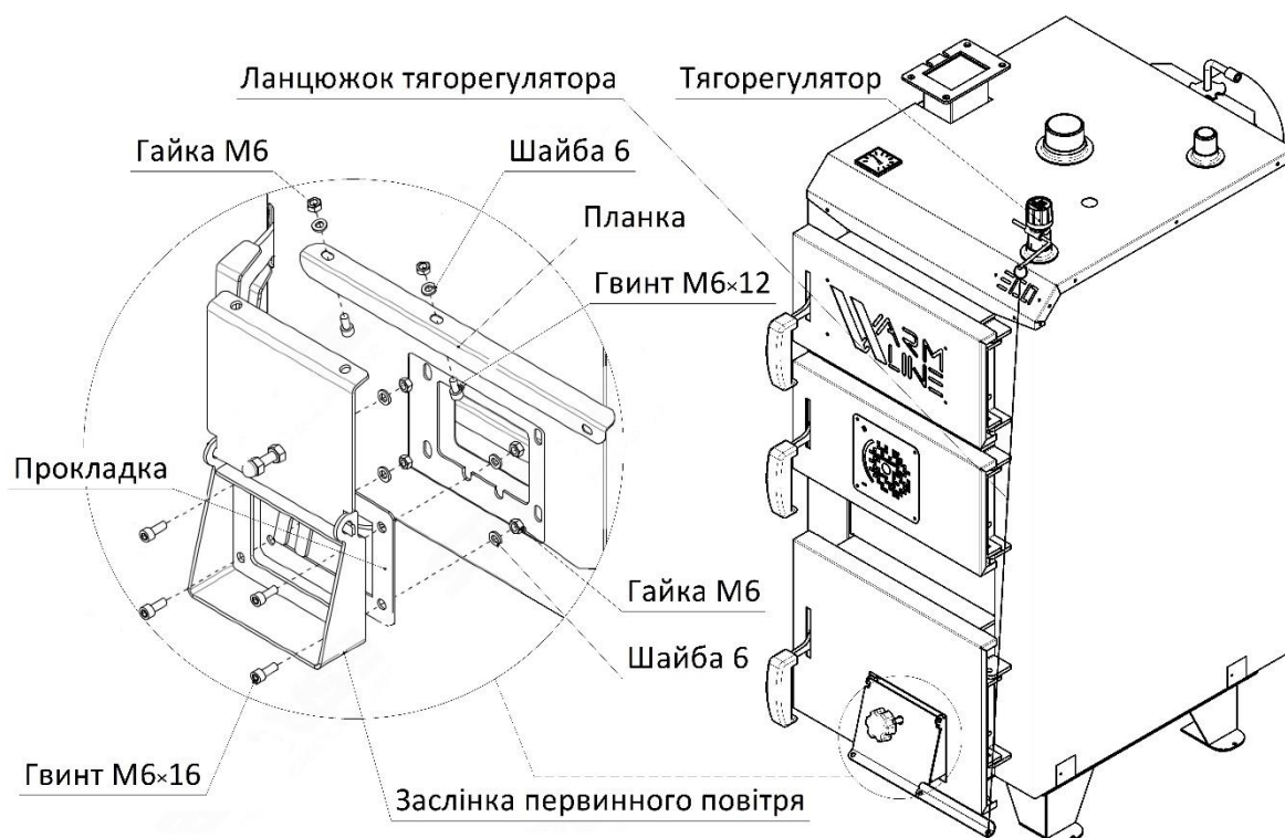
Рис. 6. Схема встановлення тягорегулятора
