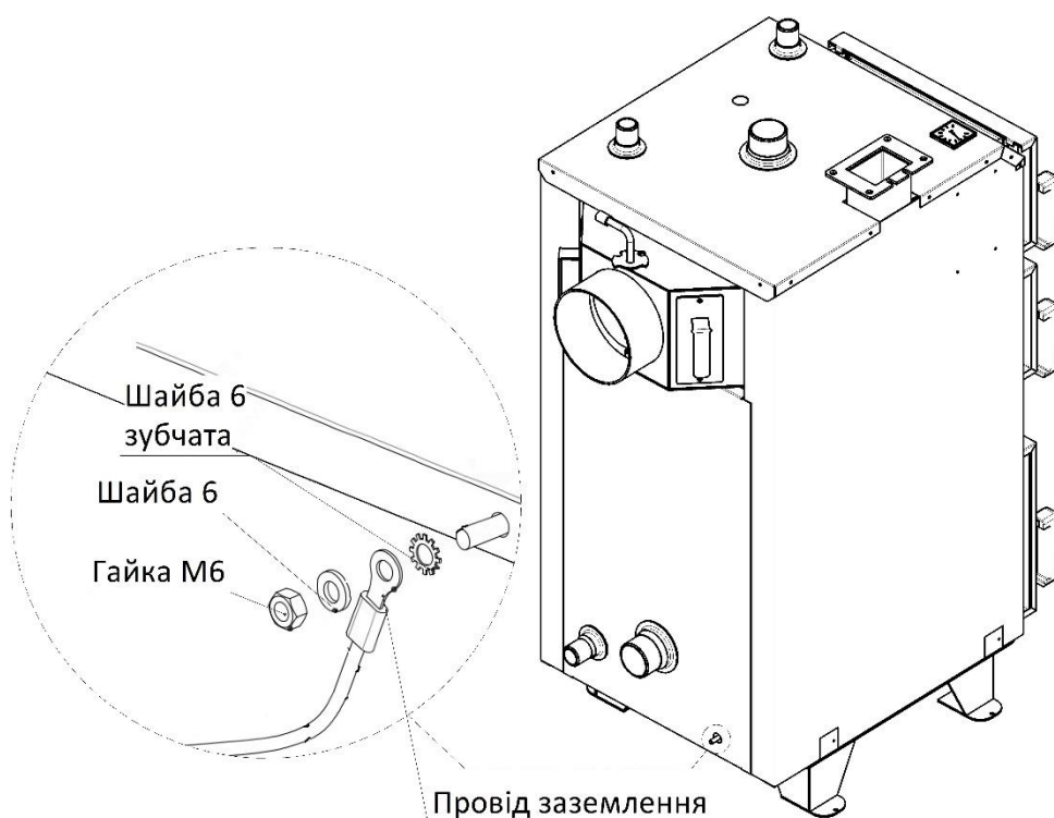
Рис. 9. Схема заземлення котла
