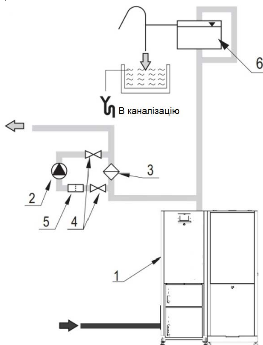
Рисунок 8 - Реалізація гравітаційного байпасу
