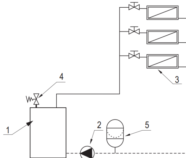
1 - джерело тепла; 2 - циркуляційний насос; 3 - контур опалення; 4 - запобіжний клапан; 5 - розширювальний бак та рекомендоване місце його установки
