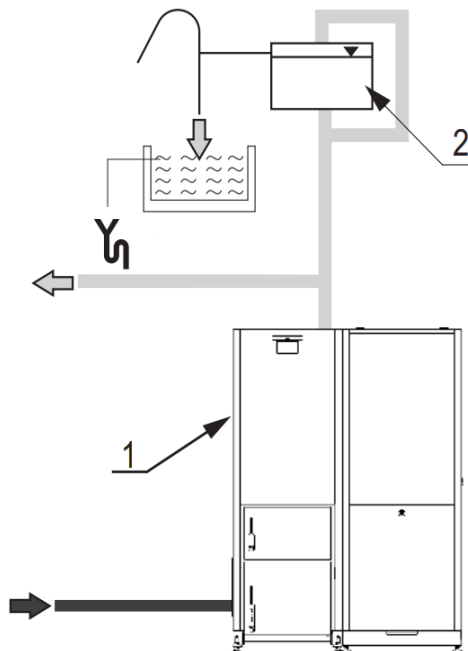
Рисунок 5 – Схема підключення розширювального баку і котла A-Pellets: 1 – котел; 2 – відкритий розширювальний бак
