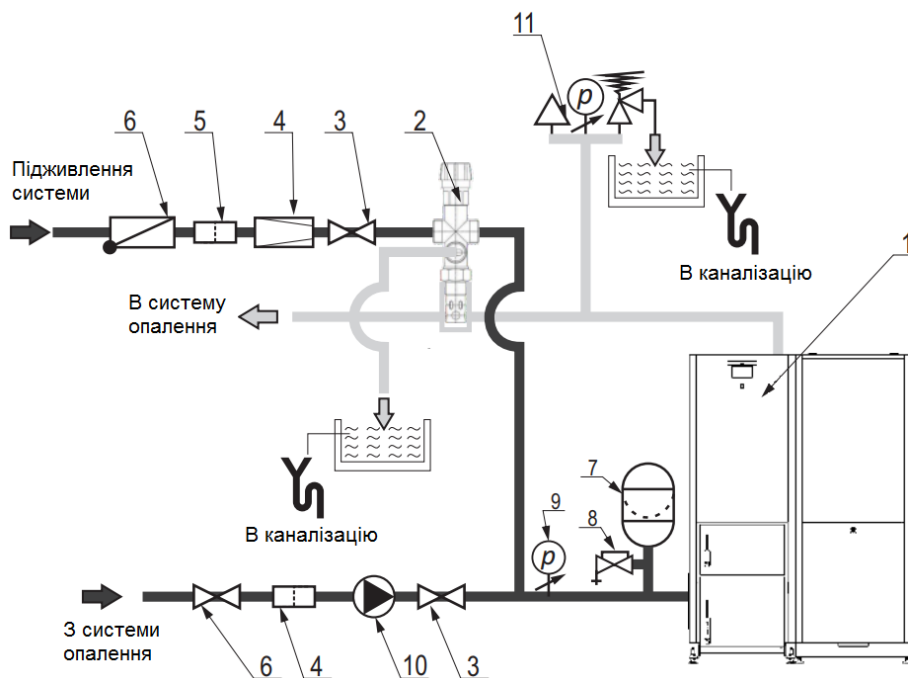
1 - котел; 2-тепловий захист від перегріву; 3-клапан кульовий; 4-редуктор тиску; 5 - фільтр питної води; 6 - зворотний клапан; 7-розширювальний бак; 8-запірний клапан; 9 - манометр; 10 - насос; 11 - група безпеки;
