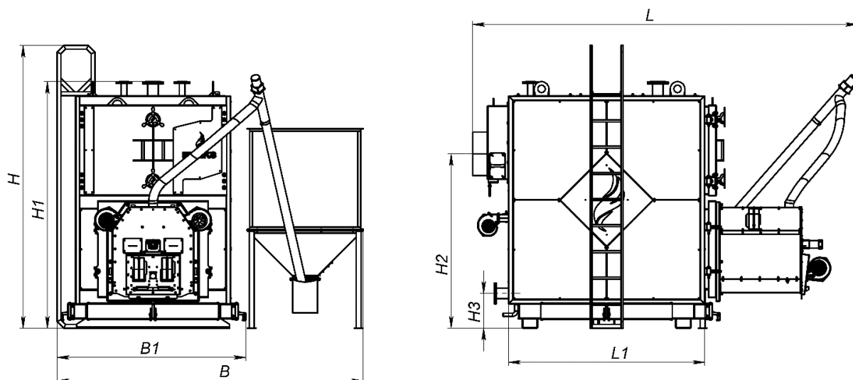
Рисунок 1 – Позначення габаритів котла
