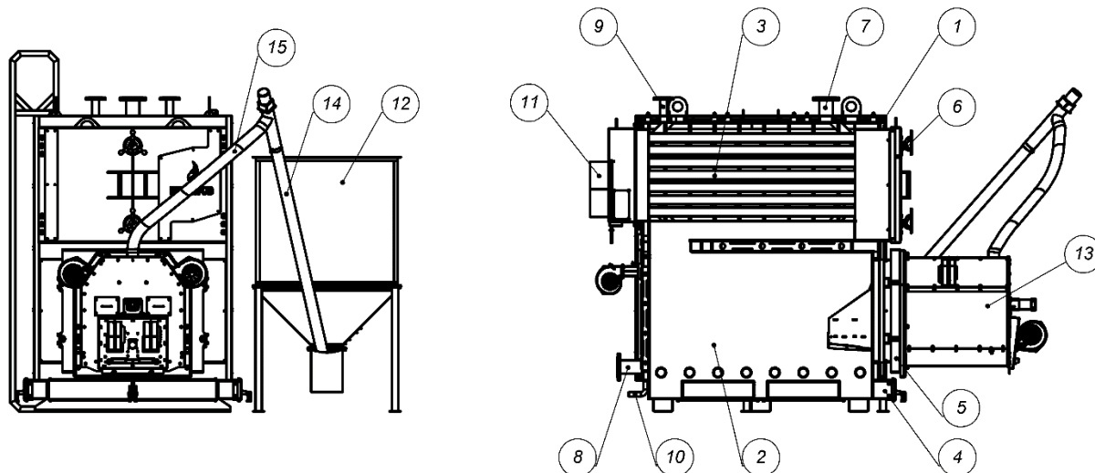
Рисунок 2 – Зовнішній вигляд та основні елементи котла
