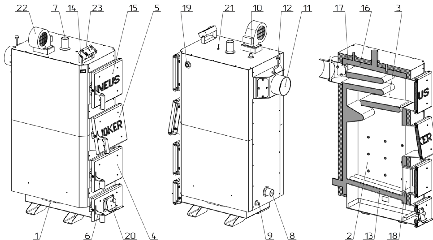
Рисунок 2 – Основні елементи котла Неус Джокер (Неус Джокер М)
