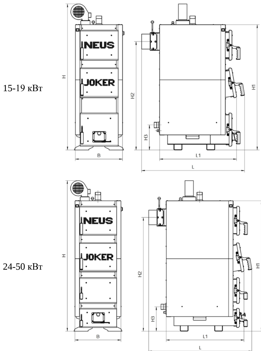
Рисунок 1 – Габаритне креслення котла Неус Джокер (Неус Джокер М)
