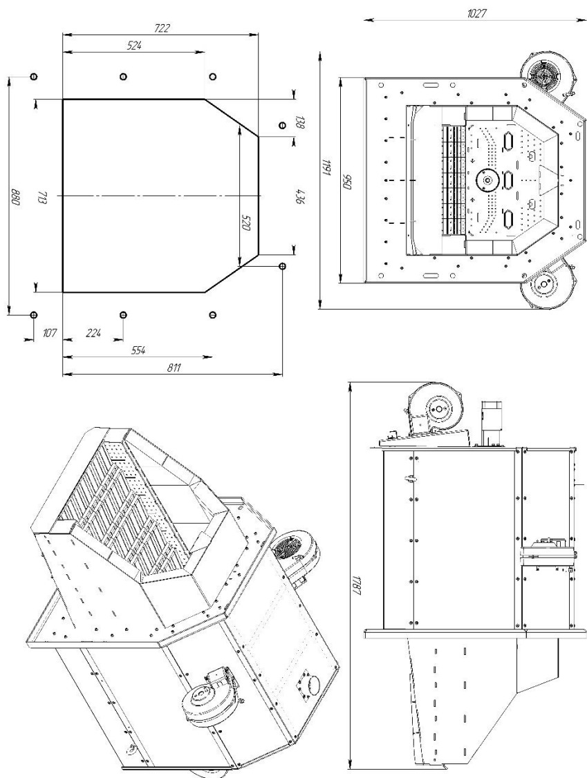
Рисунок 6.2 - Габаритные и присоединительные размеры пеллетной горелки КВТ Оптима М 800 кВт.
