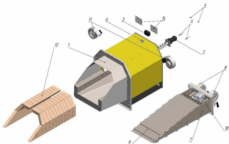
Рисунок 4.1 - Элементы конструкции горелки KVIT Optima M 800
