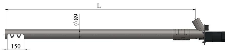
Рис.2 Геометрия комплектного шнека KVIТ Optima
