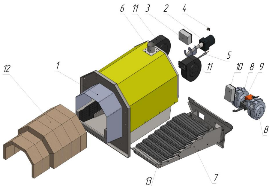
Рис.1 Элементы конструкции горелки KVIT Optima
