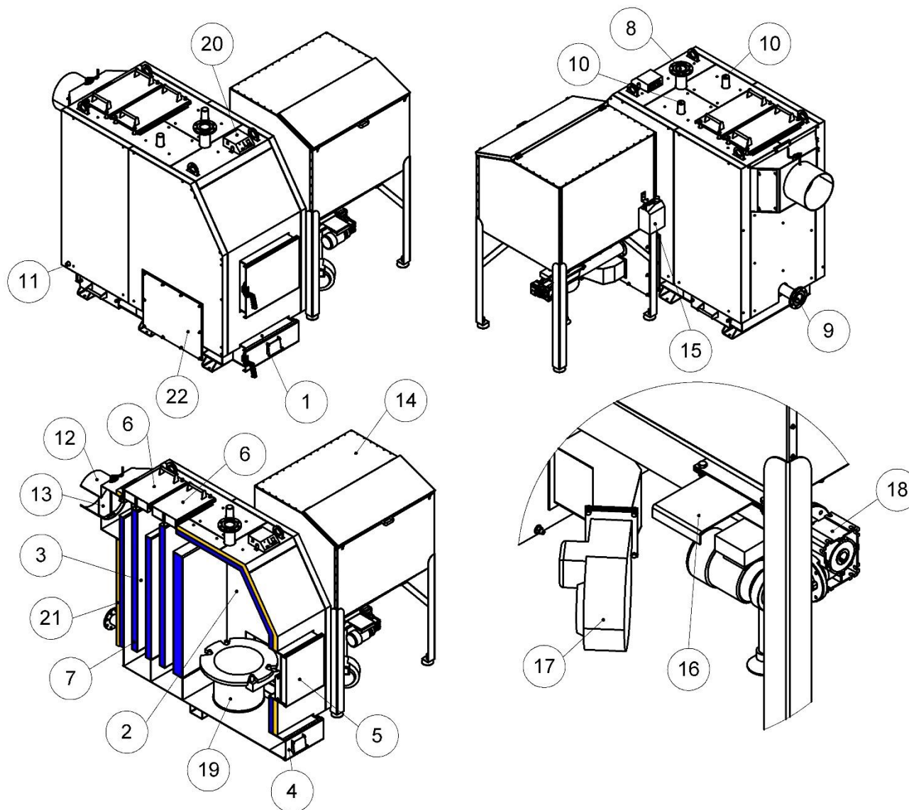
Рисунок 5.1 – Зовнішній вигляд та основні елементи котлів типу КТПк
