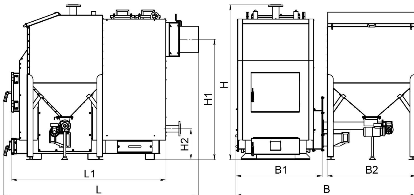
Рисунок 3.1 – Позначення габаритів котла типу КТПк
